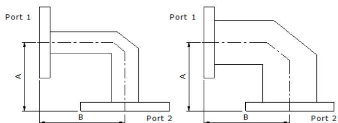
E-Plane
